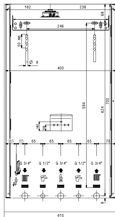
Dima di montaggio
